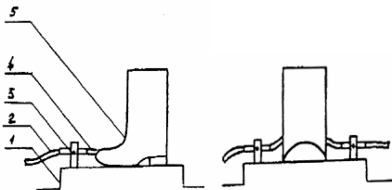
Схема установки по проверке огнезащитных свойств резиновой обуви:
