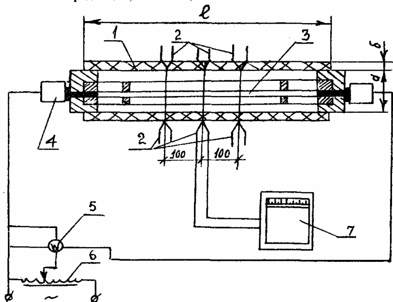
Рис. 4. Принципиальная схема установки для определения теплопроводности:
