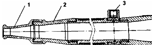
Рис. 2.1. Ствол-водомер:
