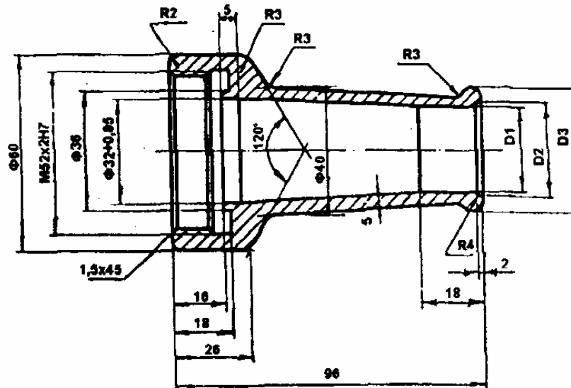
Рис. 2.1. Ствол-водомер:
