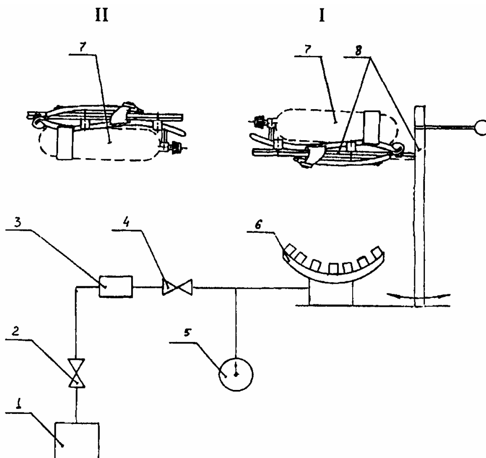
Рисунок. 3. Схема огневой установки по определению устойчивости дыхательного аппарата к воздействию пламени:
