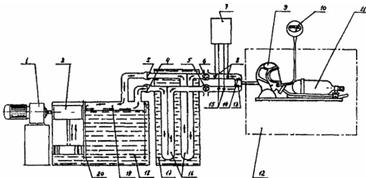
Принципиальная схема стенда-имитатора дыхания человека:
