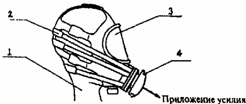
Рисунок 2. Установка для определения прочности соединения легочного автомата и основной лицевой части:
