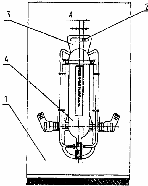
Рисунок 1. Принципиальная схема стенда для определения смещения центра массы:
