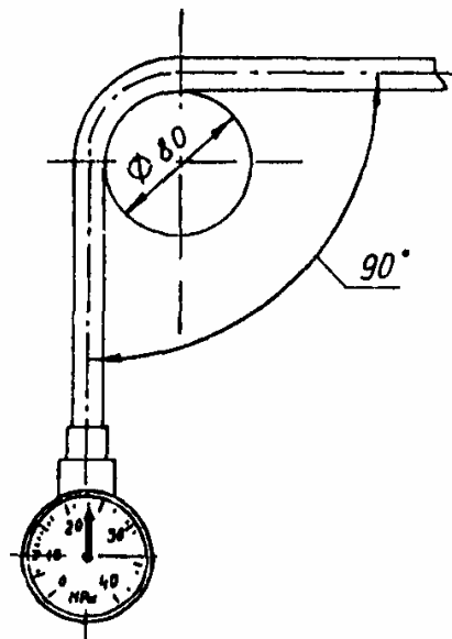
Рисунок 6. Схема определения работоспособности шланга высокого давления
