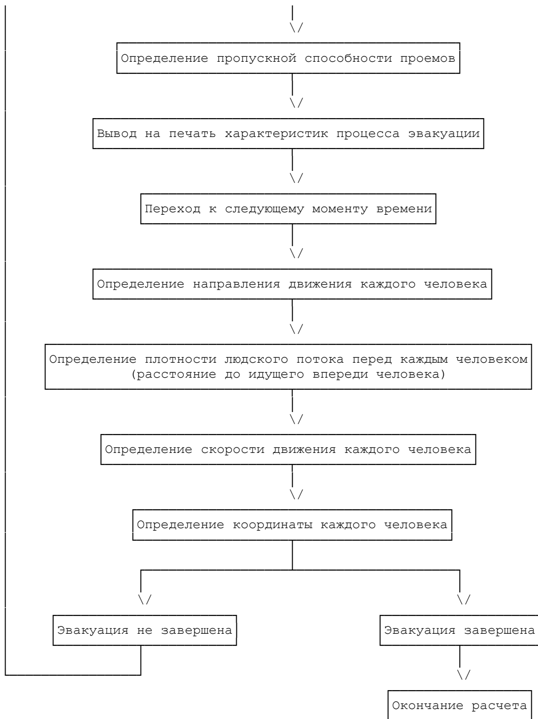
Рис. ПЗ.2. Блок-схема определения расчетного времени эвакуации людей из здания
